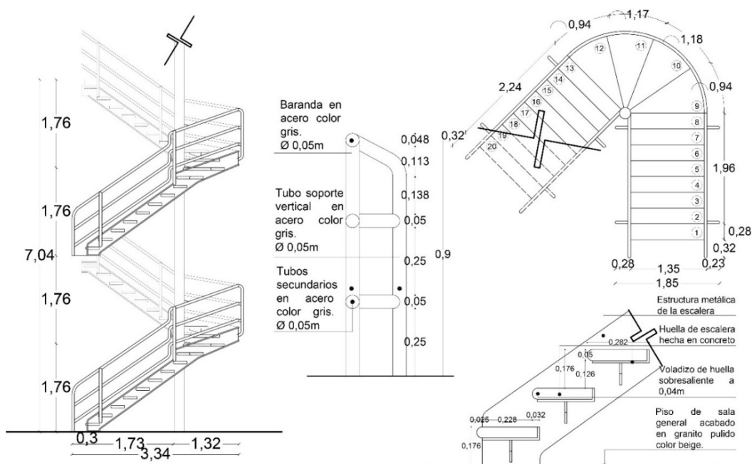
Imagen 28. Detalle de la escalera interna Biblioteca pública municipal. Fuente: Elaborada por autores de este trabajo.
