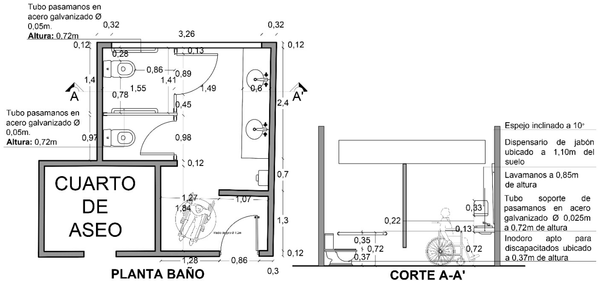
Imagen 14. Batería sanitaria de la Biblioteca Banco de la República. Fuente: Elaborada por autores de este trabajo.
