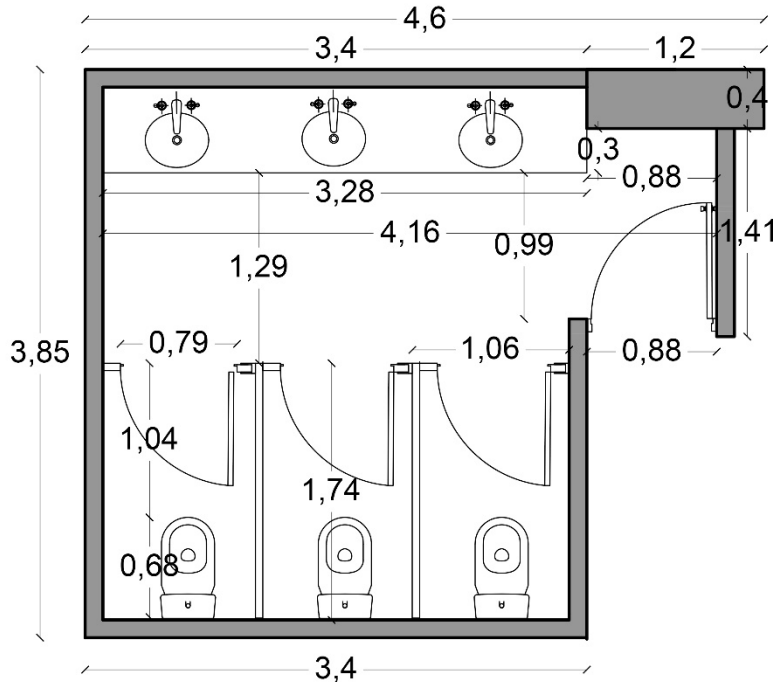
Imagen 32. Batería sanitaria de la biblioteca pública municipal. Fuente: Elaborada por autores de este trabajo.
