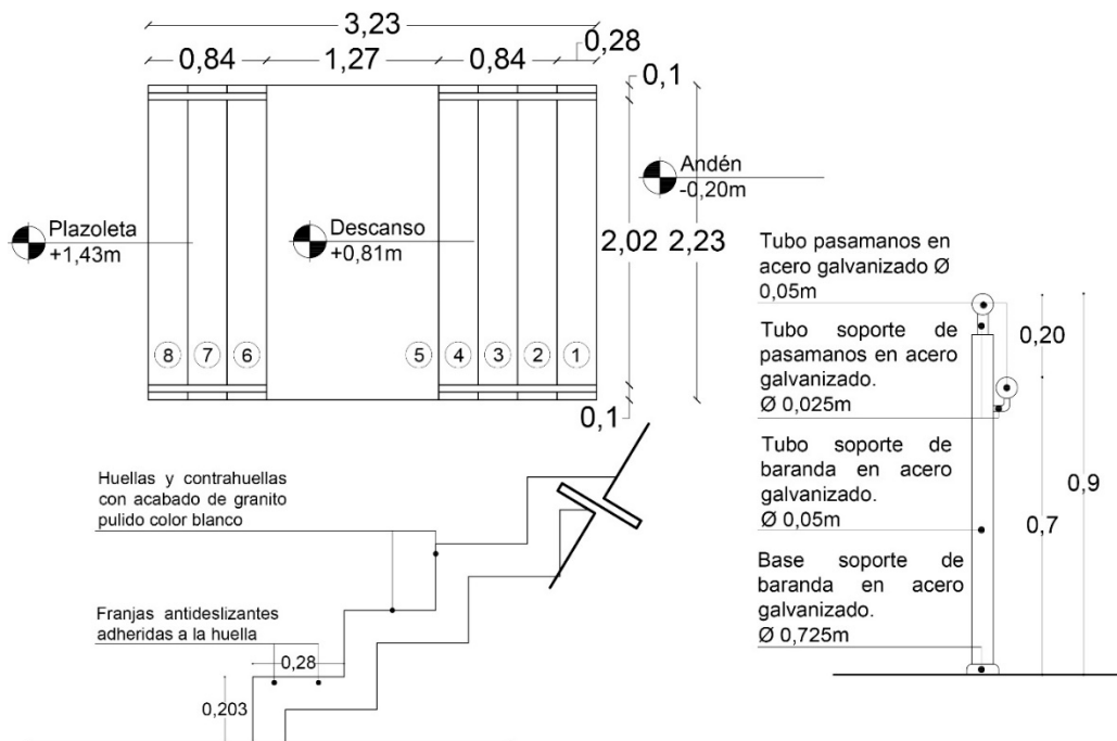
Imagen 12. Detalle de la escalera externa Biblioteca Banco de la República. Fuente: Elaborada por autores de este trabajo.
