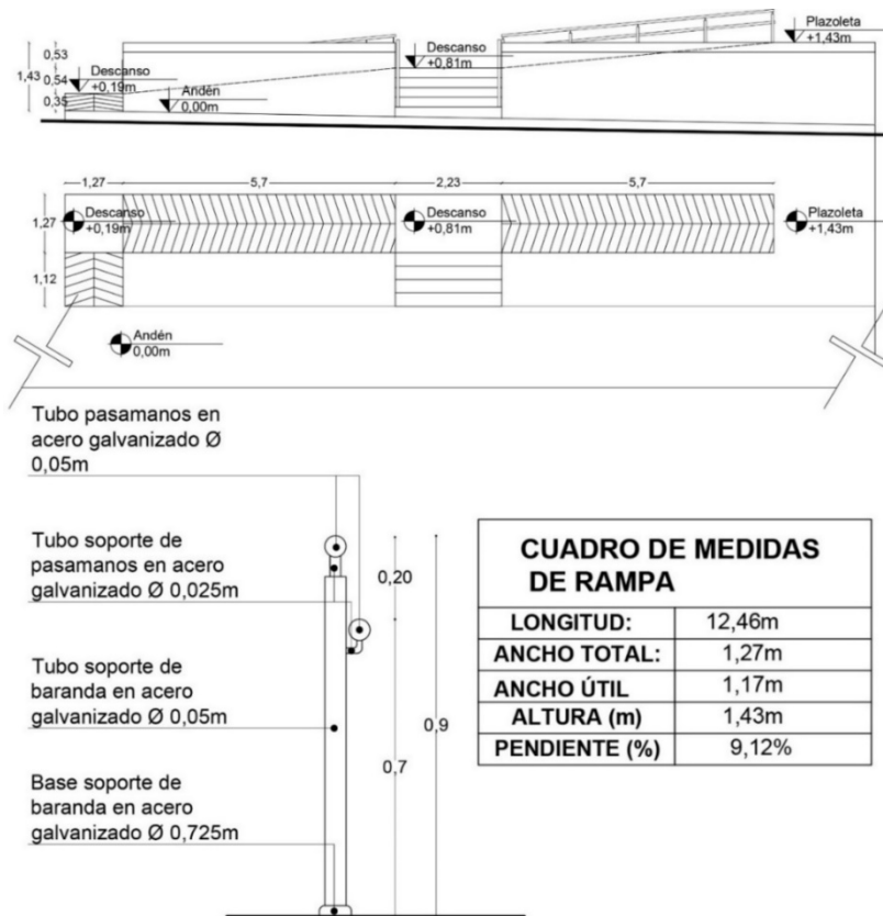
Imagen 13. Detalle de la rampa de la Biblioteca Banco de la República. Fuente: Elaborada por autores de este trabajo.
