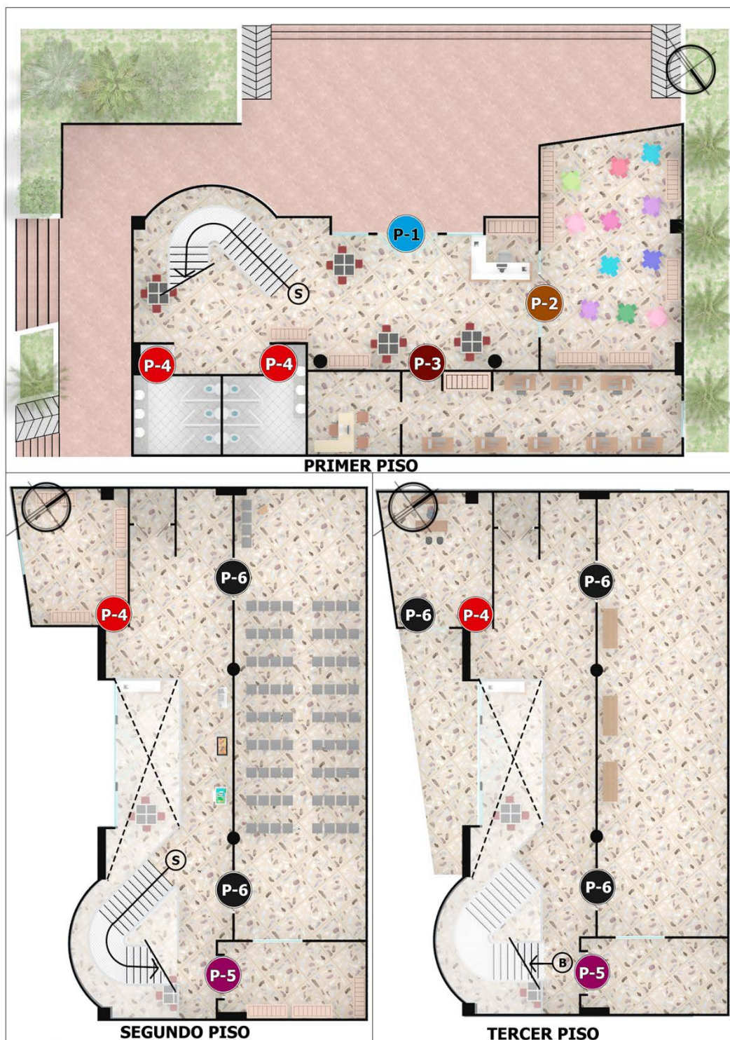
Imagen 27. Plano de puertas y ventanas de la Biblioteca pública municipal de Sincelejo. Fuente: Elaborada por autores de este trabajo.
