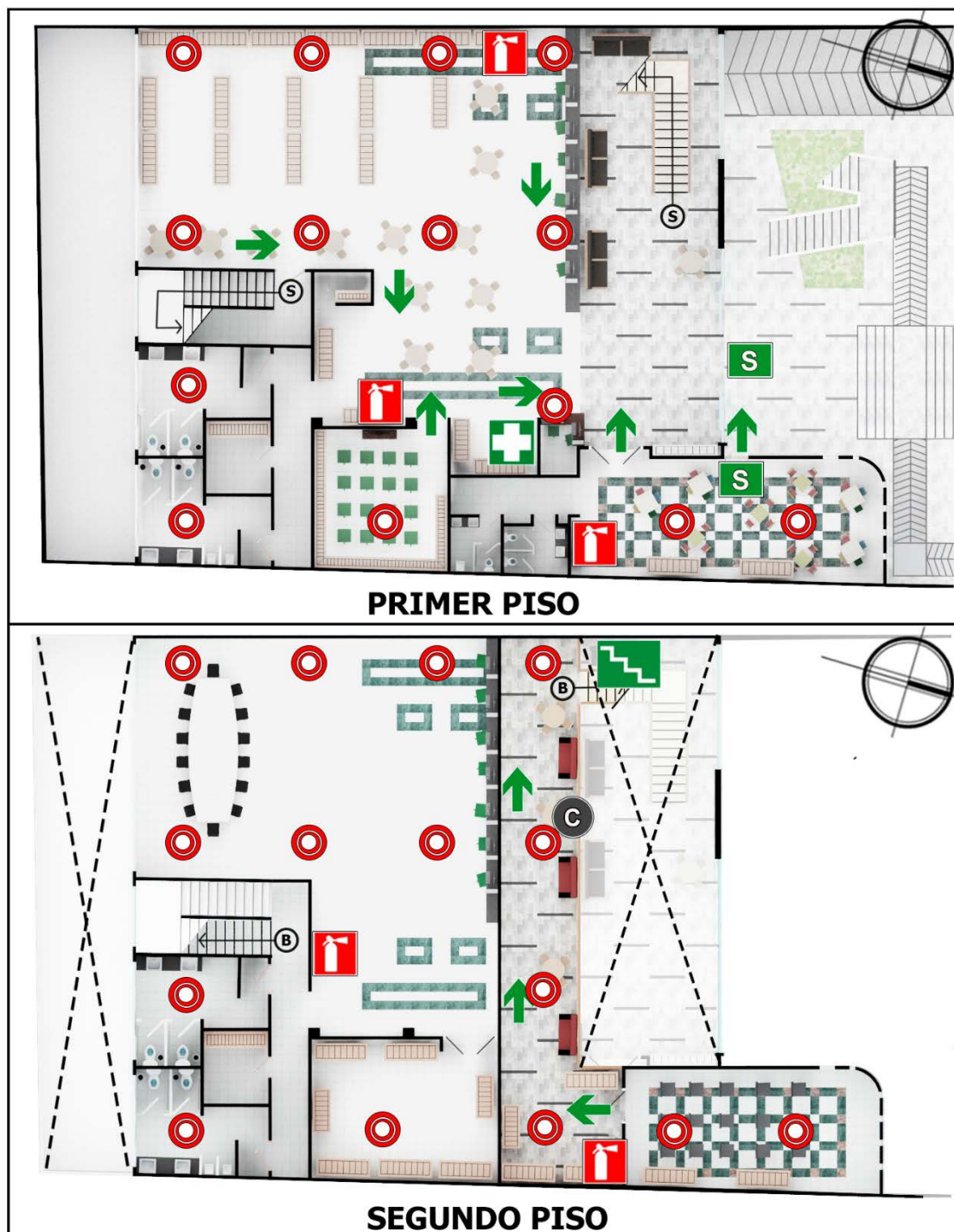
Imagen 16. Medidas de protección contra incendios de la Biblioteca Banco de la República. Fuente: Elaborada por autores de este trabajo.
