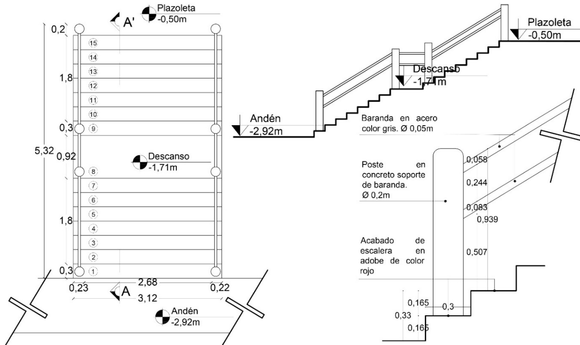
Imagen 29. Detalle de la escalera externa de la biblioteca pública municipal. Fuente: Elaborada por autores de este trabajo.
