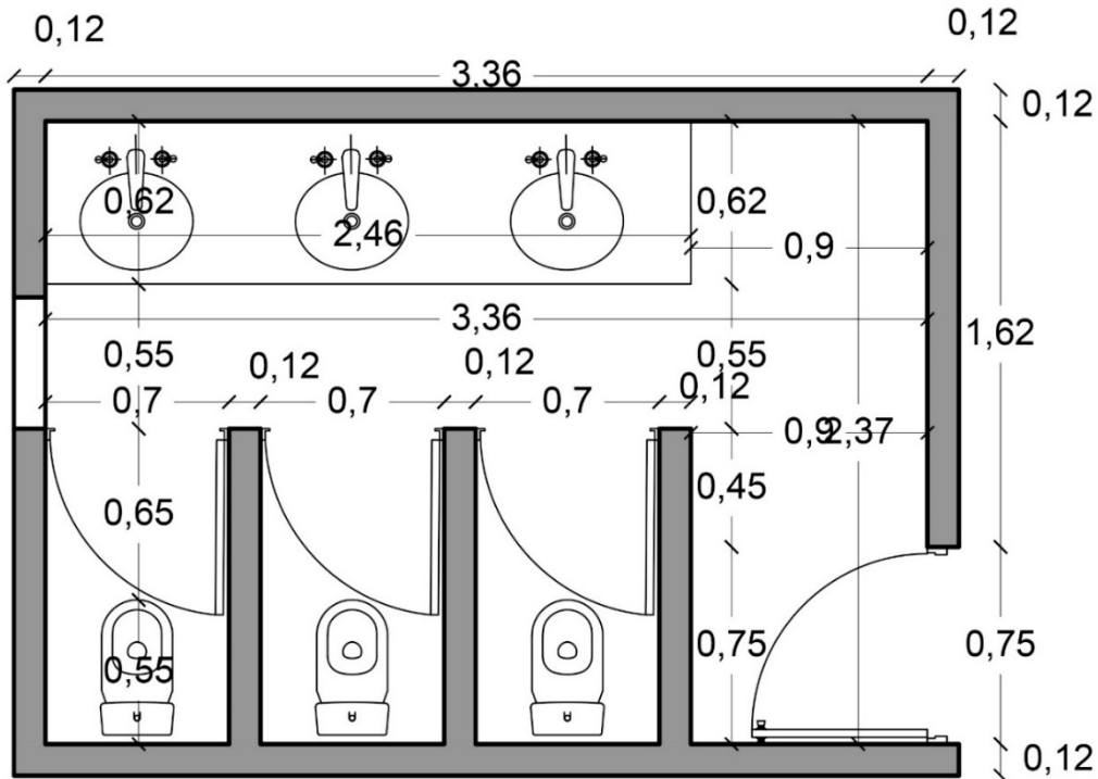
Imagen 22. Batería sanitaria de la Biblioteca pública departamental. Fuente: Elaborada por autores de este trabajo
