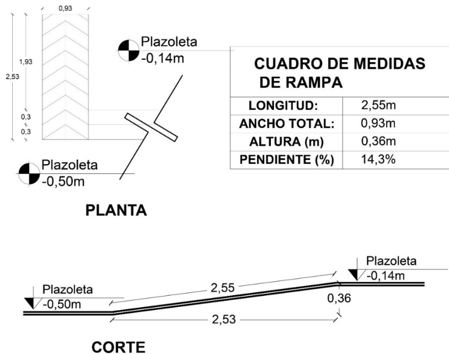
Imagen 31. Plano de detalle de rampa de la Biblioteca pública municipal. Fuente: Elaborada por autores de este trabajo.
