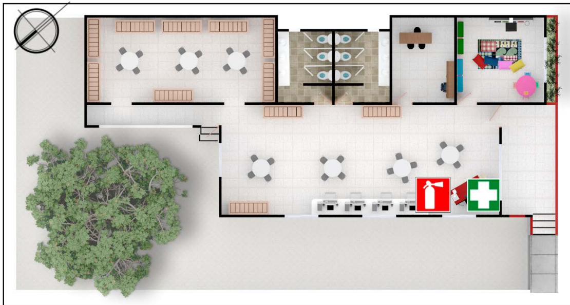
Imagen 23. Plano de medidas de protección contra incendios de la Biblioteca pública departamental. Fuente: Elaborada por autores de este trabajo.
