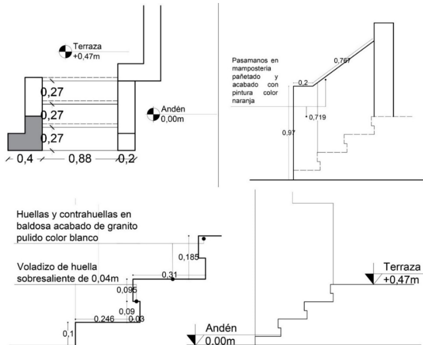
Imagen 21. Detalle de la escalera externa Biblioteca pública departamental. Fuente: Elaborada por autores de este trabajo.
