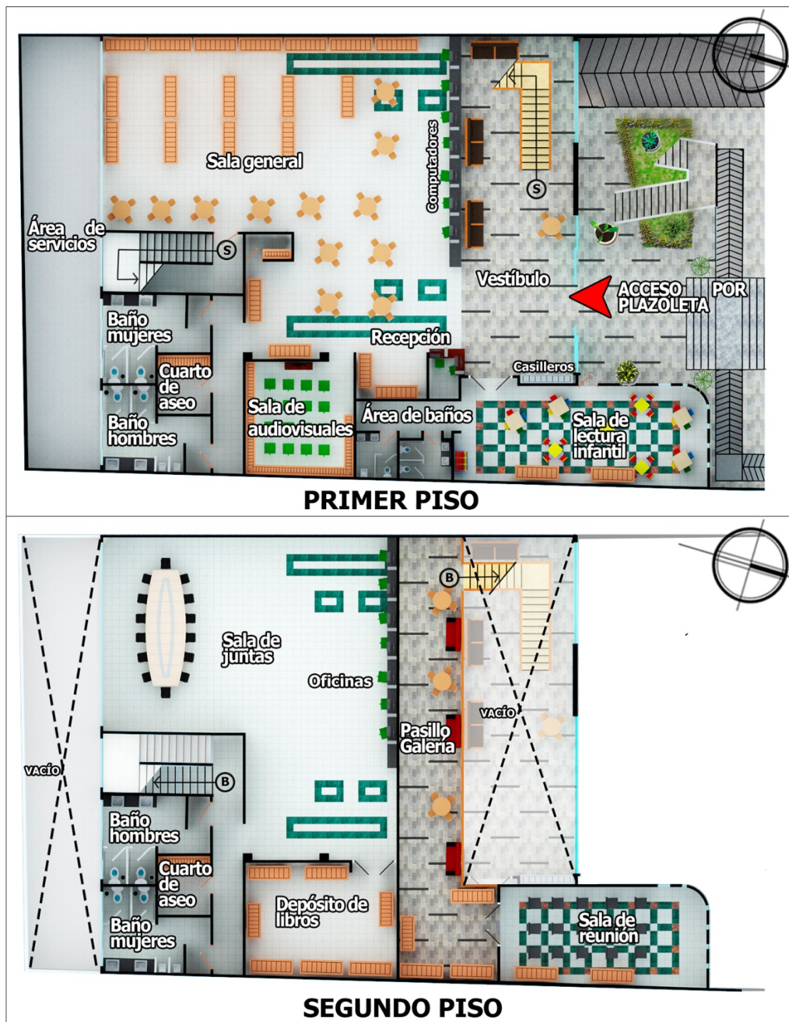
Imagen 7. Plantas de la Biblioteca Banco de la República. Fuente: Elaborado por autores de este trabajo
