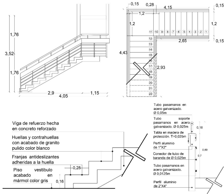
Imagen 11. Detalle de la escalera interna Biblioteca Banco de la República. Fuente: Elaborada por autores de este trabajo.
